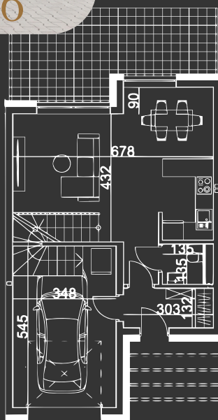
Rzut parteru
