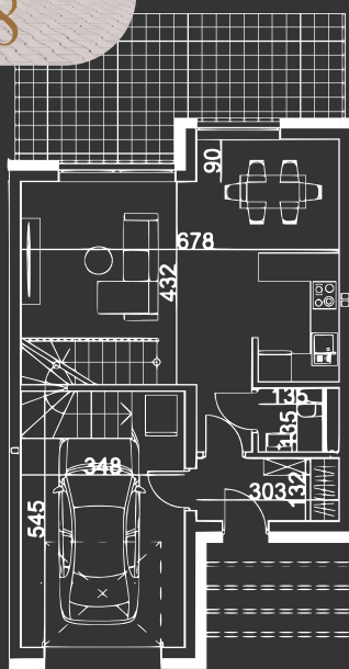
Rzut parteru
