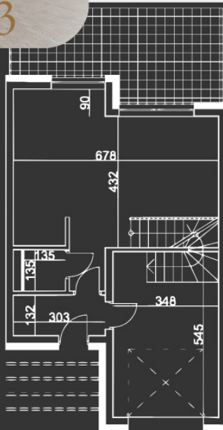
Rzut parteru
