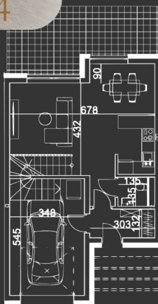
Rzut parteru
